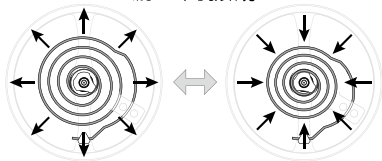
游丝的振荡
